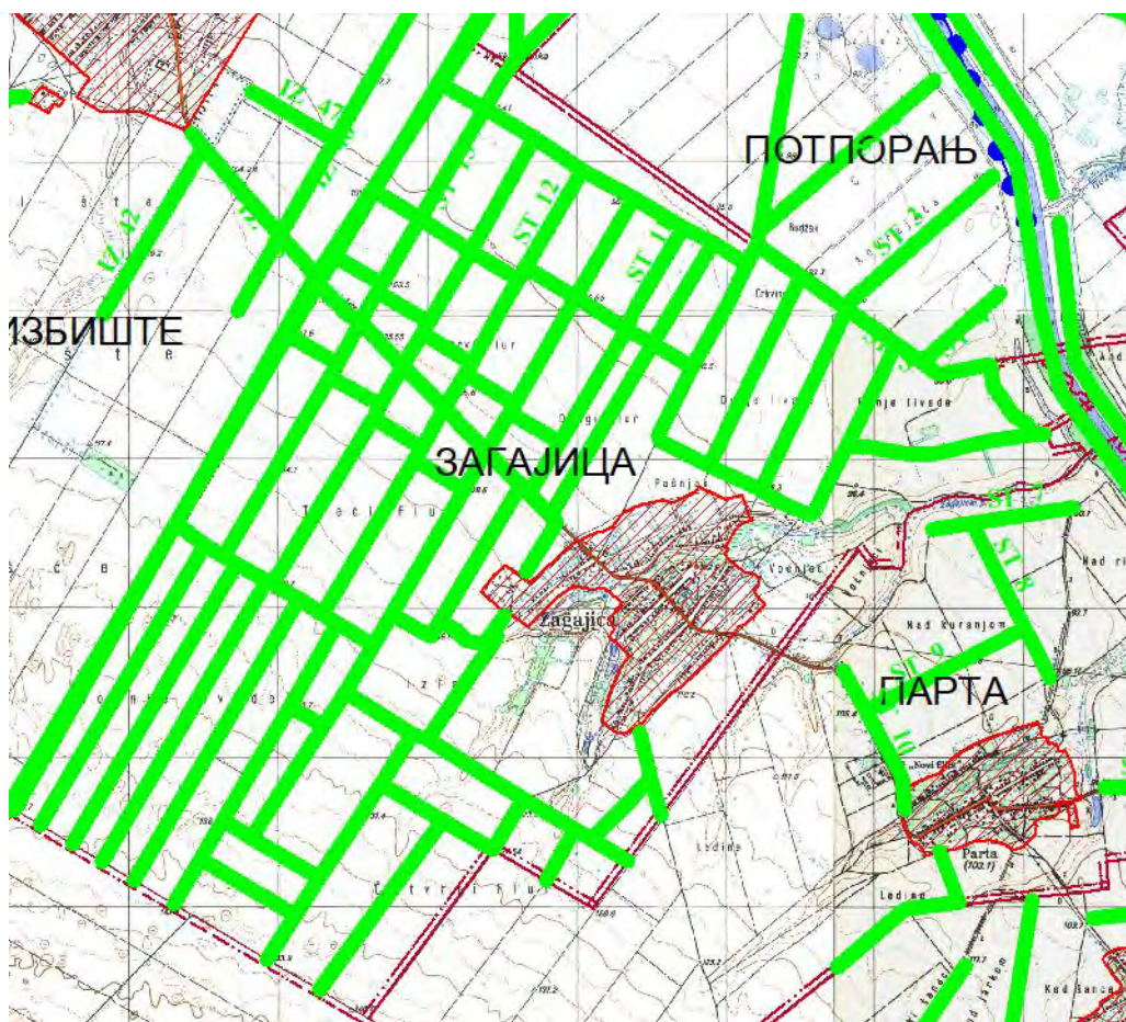
Слика 9: Предлог мрже пољозаштитних појасева у КО Загајица
