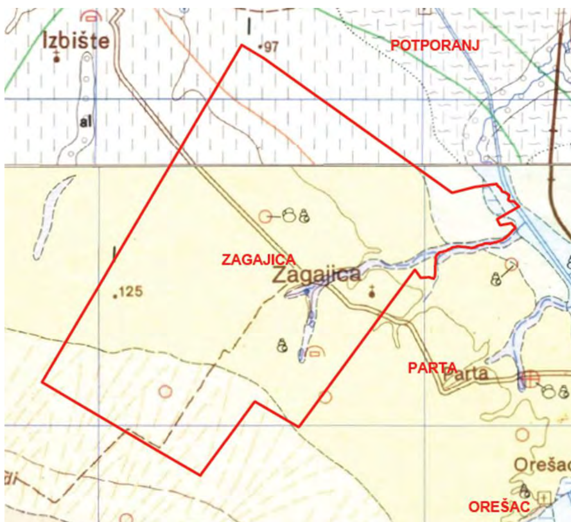
Слика 4: Геолошка карта КО Загајица
