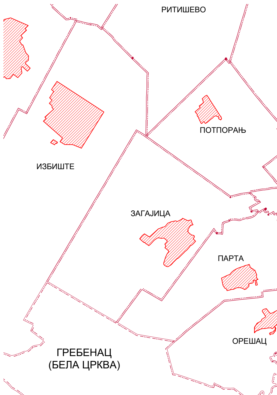
Слика 12: Подручје града Вршца и положај катастарских општине Загајица
