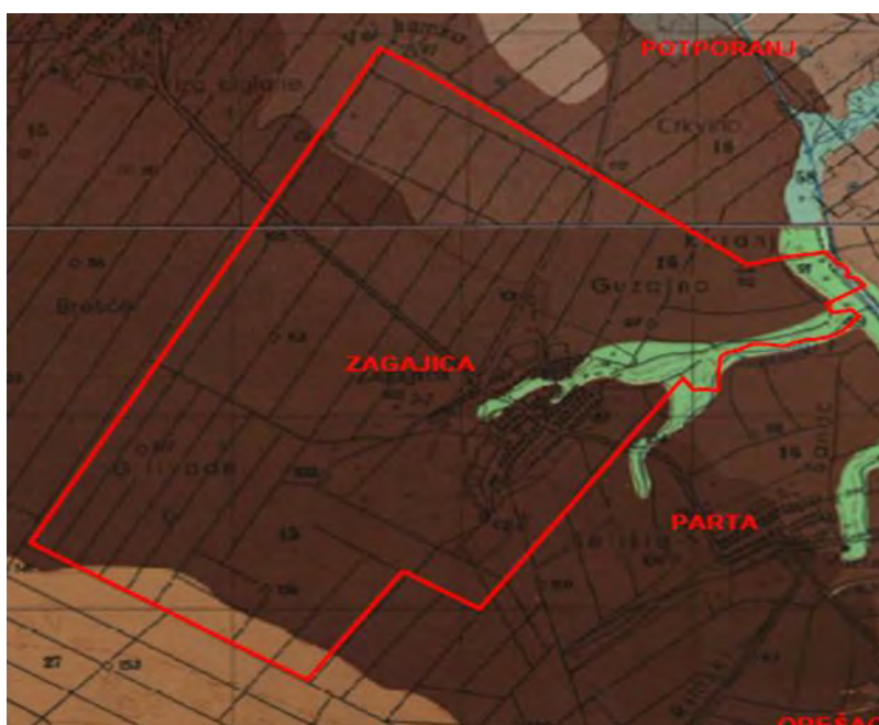
Слика 7: Педолошка карта КО Загајица
